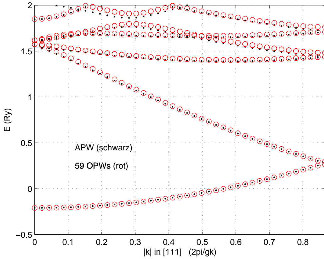
ELEKTRON-Bandstruktur fcc Al APW 12-5-2009
